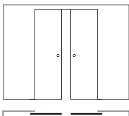
Edisse SYNTESIS®LINE dvojkřídlové | 22-25
