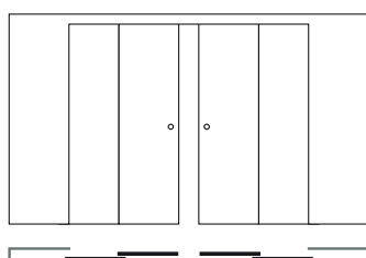
Edisse TELESKOPICKÉ dvojitě | 30-31
